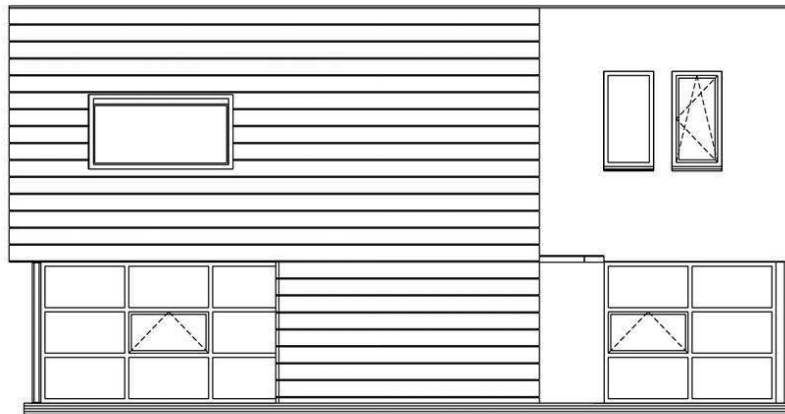
Voorgevel villa, gebouw 1 en 4
