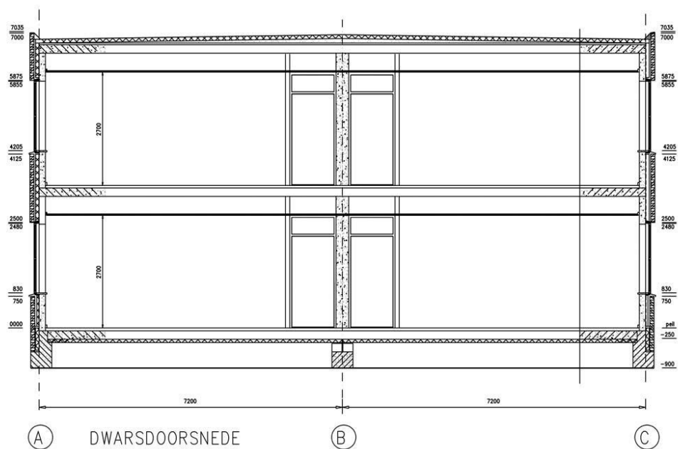
Dwarsdoorsnede 2/1 kap, gebouw 2 voorzijde
