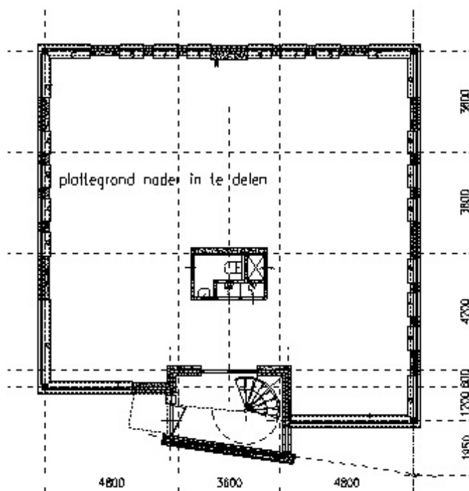
Plattegrond villa, begane grond, gebouw 3 en 4 gesp.
