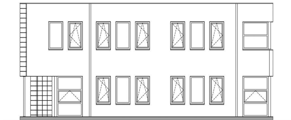
Zijgevel villa
