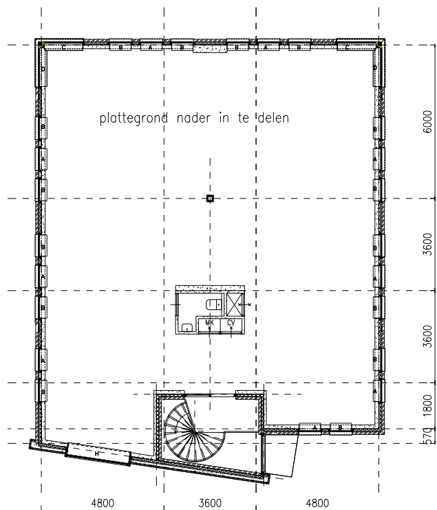
Plattegrond villa+, verdieping, gebouw 1 en 5 gesp.
