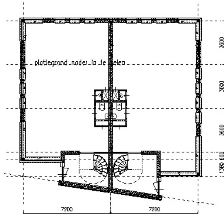
Plattegrond 2/1 kap, begane grond, gebouw 2
