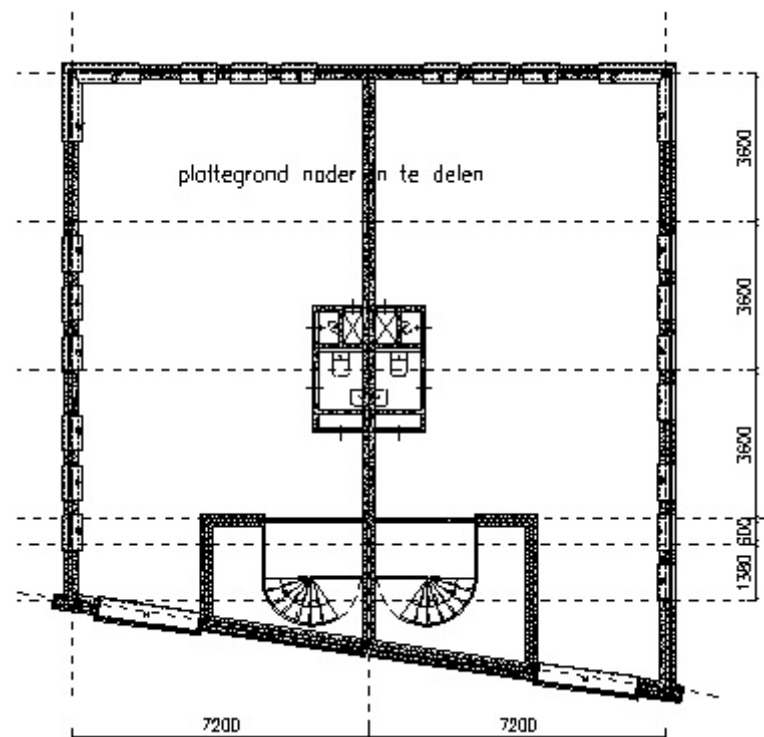
Plattegrond 2/1 kap, verdieping, gebouw 2
