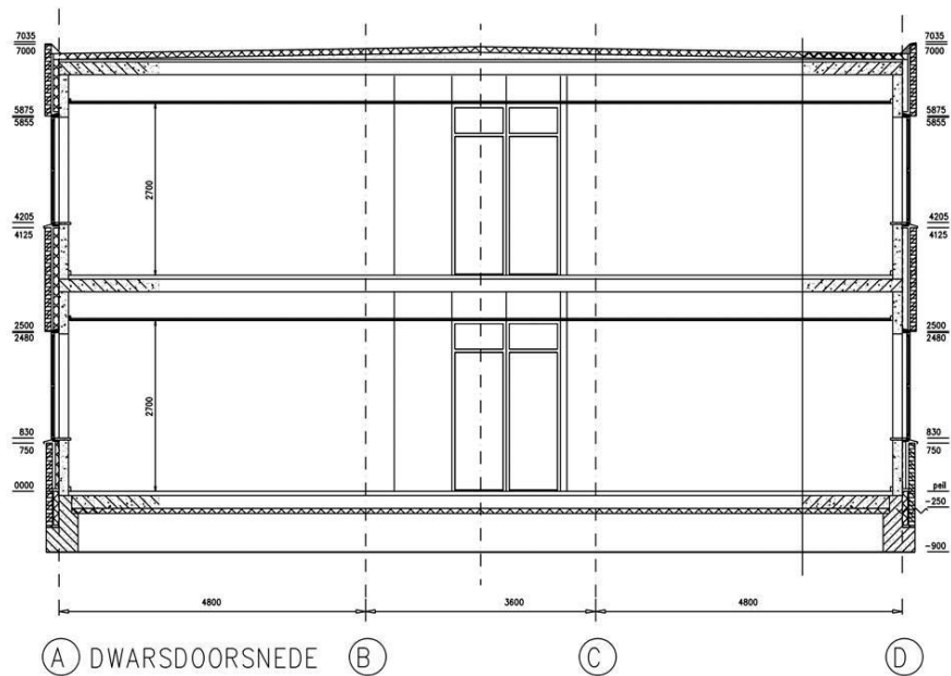
Dwarsdoorsnede villa, gebouw 1, 3 gesp., 4 en 5 gesp. voorzijde
